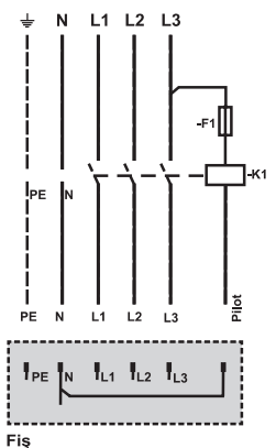
Standart Kilit Mekanizması
