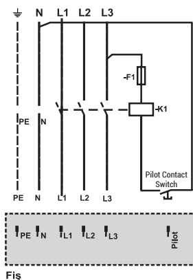
Pilot Kilit Mekanizması
