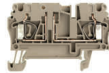
ZTR 2.5/0.TNHE
